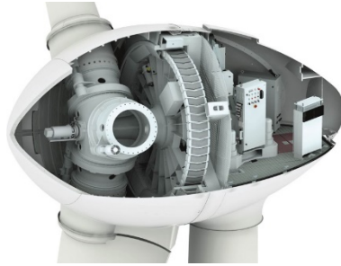
Abbildung 9: Gondelschnitt des getriebelosen Antriebssystems der ENERCON E-53
