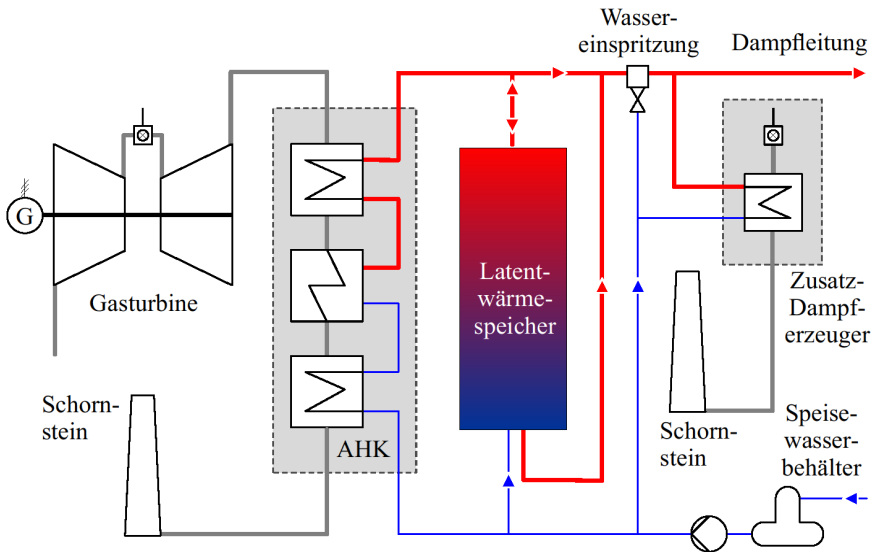
Abbildung 2: Verfahrenstechnische Einbindung des Speichers im Heizkraftwerk Wellesweiler
