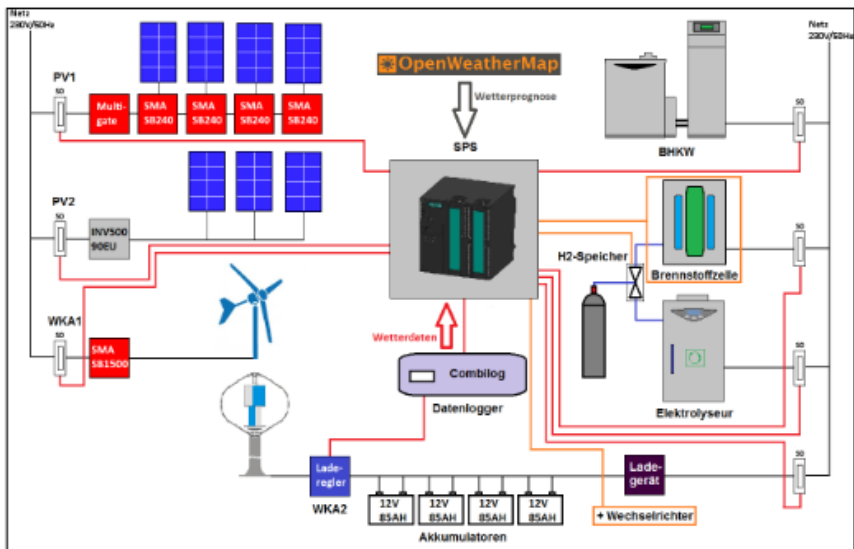
Bild 1: Übersicht des Aufbaus des virtuellen Kraftwerkes
