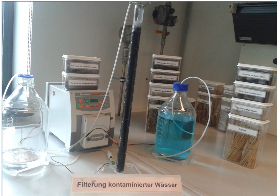
Abbildung 4: Biokohle als Filtermaterial in einer Säule zur Reinigung gefärbten Wassers 13
