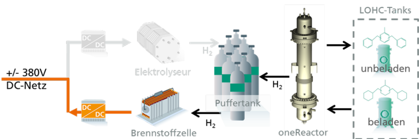
Abbildung 6: Prozess der Ausspeicherung von Energie aus dem LOHC-Container
