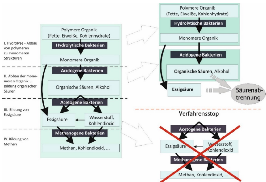
Abbildung 1: Biogasbildung mit vier Phasen des anaeroben Abbaus (links), Gewinnung organischer Säuren mit zwei Phasen des anaeroben Abbaus (rechts)
