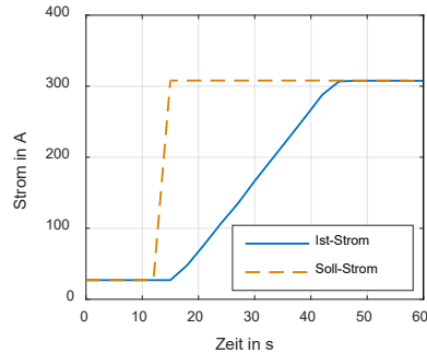
Abbildung 5: Lastwechsel des Elektrolyseurs von 27 A auf über 300 A
