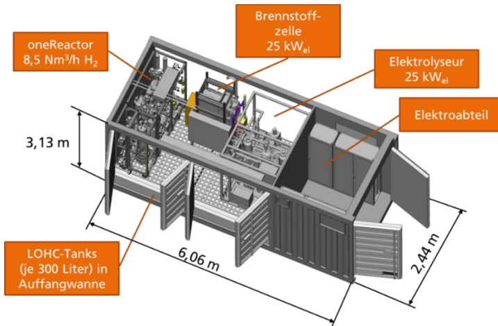
Abbildung 2: Vereinfachte Darstellung des LOHC-Containers am Fraunhofer IISB
