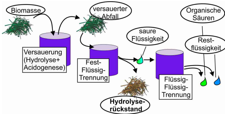
Abbildung 2: Schema des verfahrenstechnischen Ablaufs zur Erzeugung organischer Säuren aus Biomasse mit der Kenntlichmachung des Hydrolyserückstandes
