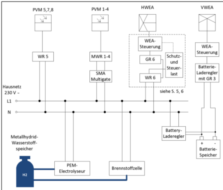
Bild 2: Übersicht Systemaufbau des virtuellen Kraftwerkes
