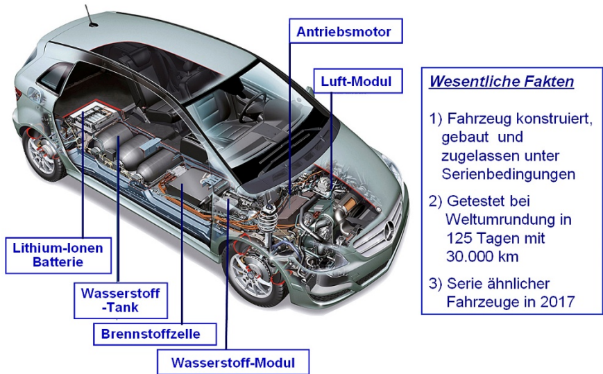
Abb. 6: Daimler B-Klasse mit H 2 -Speicherung (700b) und Brennstoffzelle
