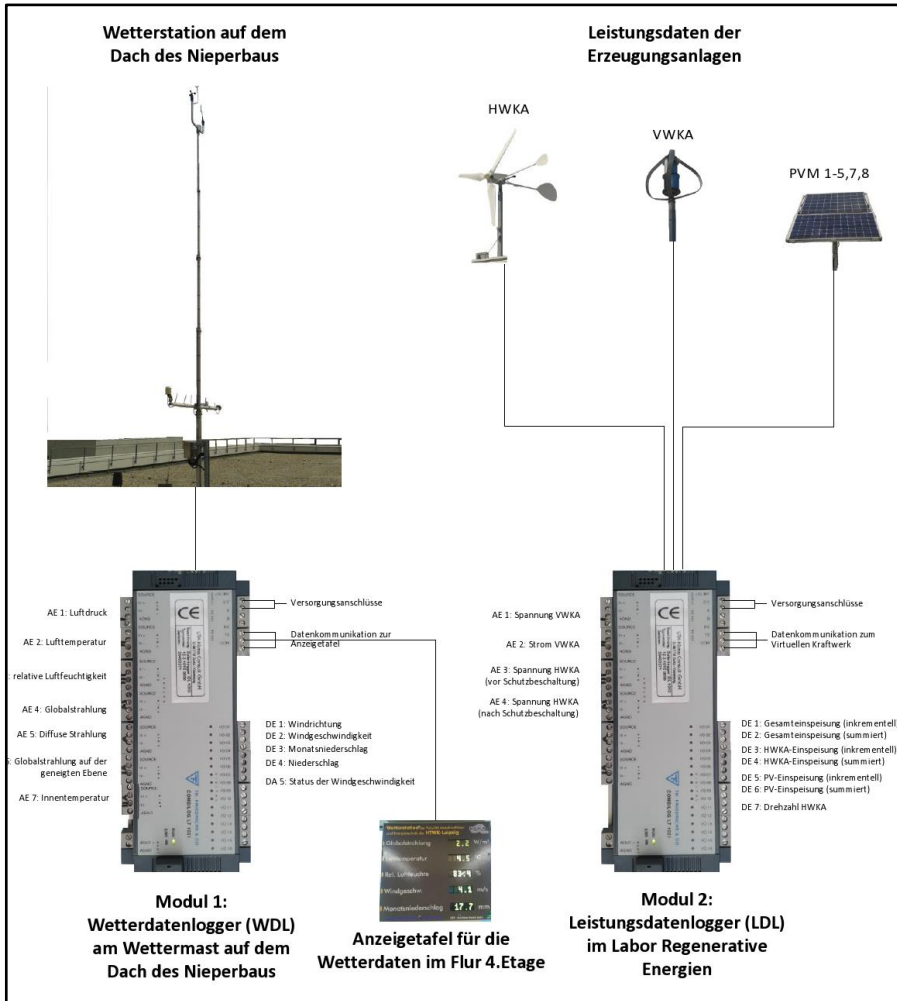
Bild 3: Schema für die Erfassung der meteorologischen Daten und der Leistungsdaten
