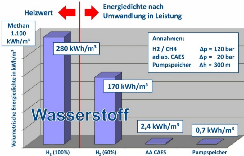
Abb. 3 Vergleich der Nettospeicherkapazitäten (Quelle KBB-UT) (CAES = Compressed Air Energy Storage)
