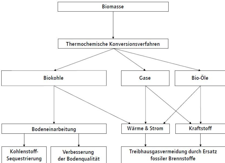
Abbildung 3: Flussdiagramm Biokohle 6
