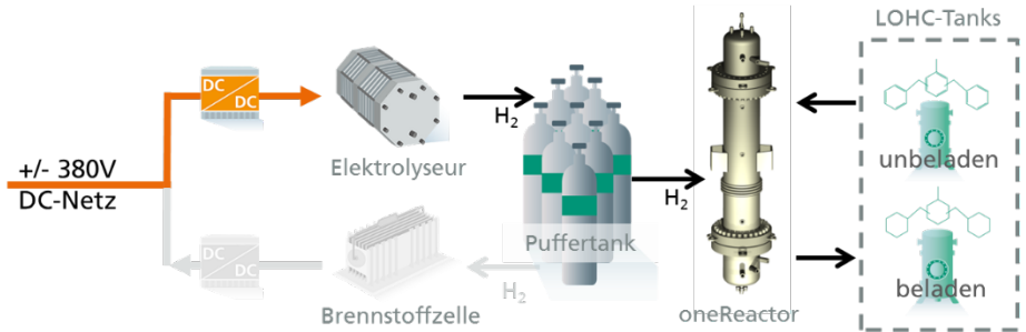
Abbildung 3: Prozess der Einspeicherung von Energie in den LOHC-Container
