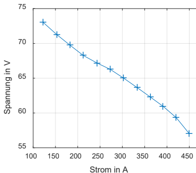
Abbildung 7: Gemessene U-I-Kennlinie der Brennstoffzelle
