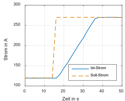
Abbildung 8: Lastwechsel der Brennstoffzelle von 120 A auf 270 A
