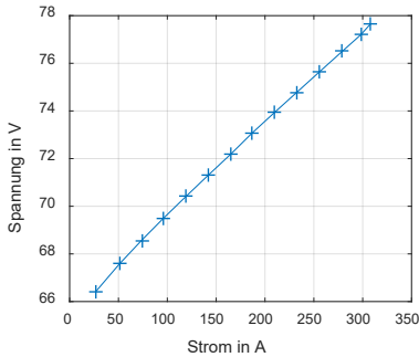
Abbildung 4: Gemessene U-I-Kennlinie des Elektrolyseurs
