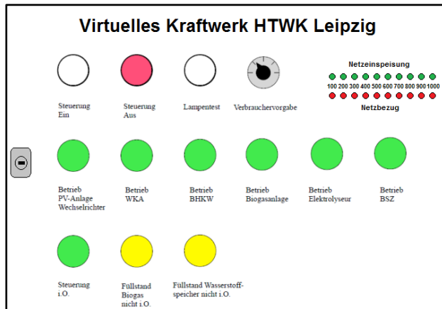
Bild 4: Bedienelemente des virtuellen Kraftwerkes
